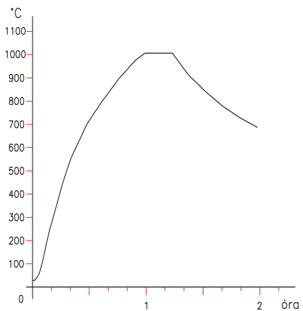
K 28/1100 tip kemence felfűtési és lehűlési diagrammja
