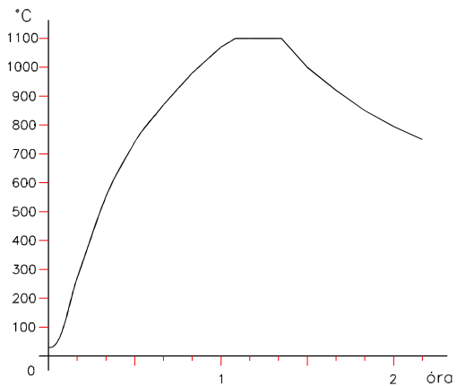
K14/1200 típusú kemence felfűtési és lehűlési diagramja
